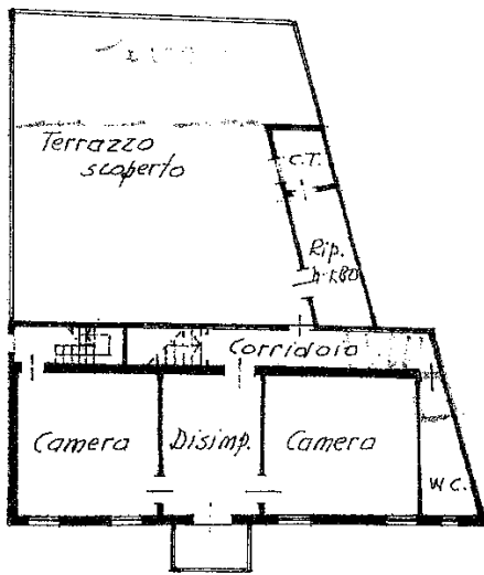
piano primo h.2.80
